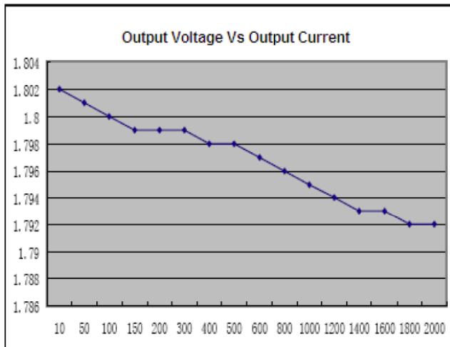
Vin=3.6V, Vout=1.8V
