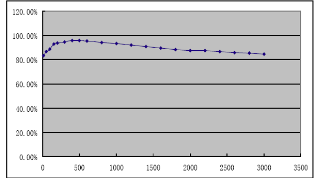
Vin=5V, Vout=3.3V
