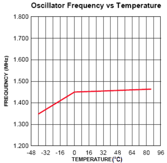
Vin=5V, Vout=3.3V
